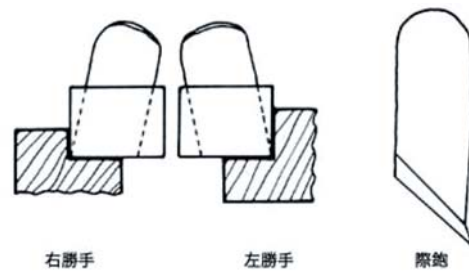
▲ 際鉋
